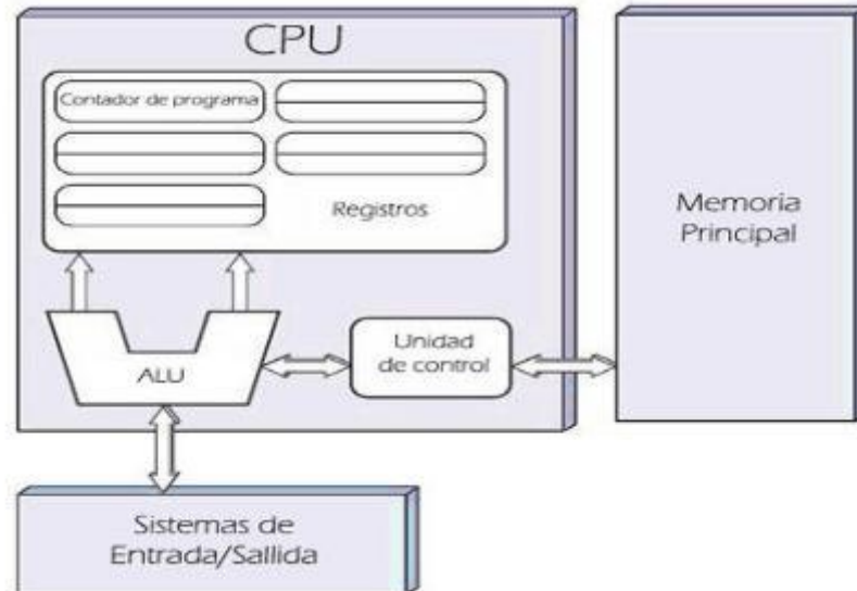
Figura 3. Arquitectura Modelo de Von Neumann
